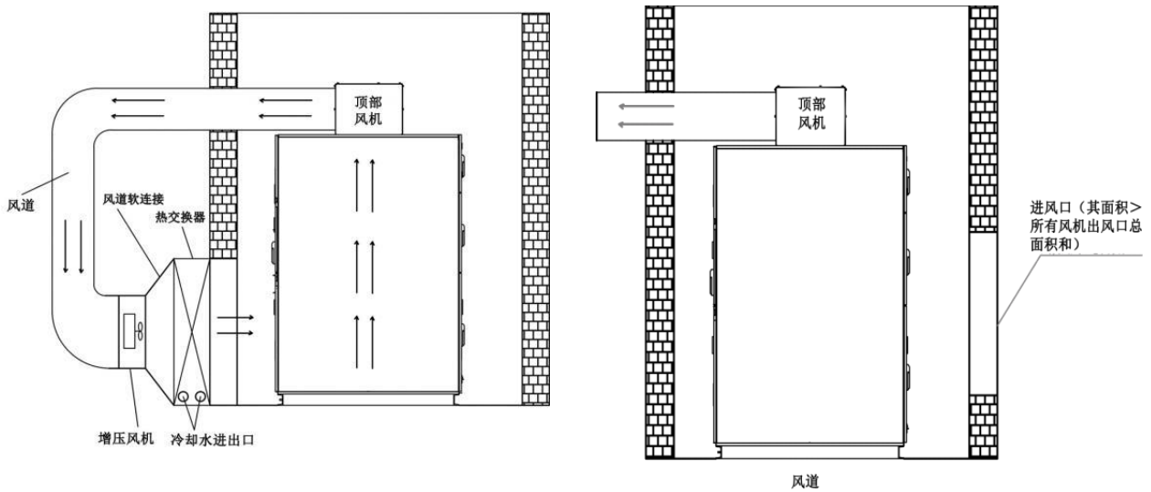
图7.5 空水冷图
