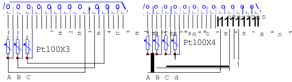
D/E/F型三路插头内部示意图
