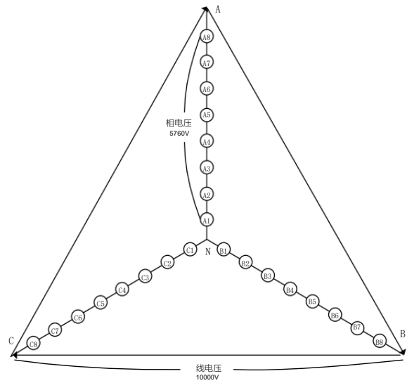
图3.4 10kV变频器单元电压叠加图
