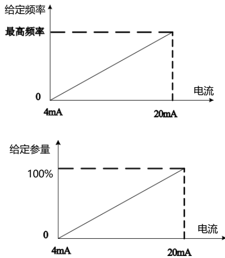
图5.22 模拟给定
