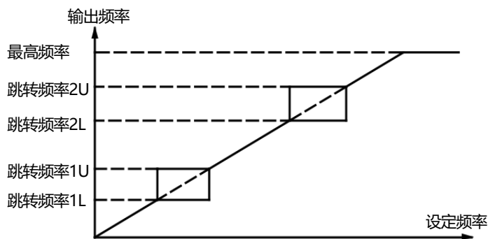
图5.24 跳转频率
