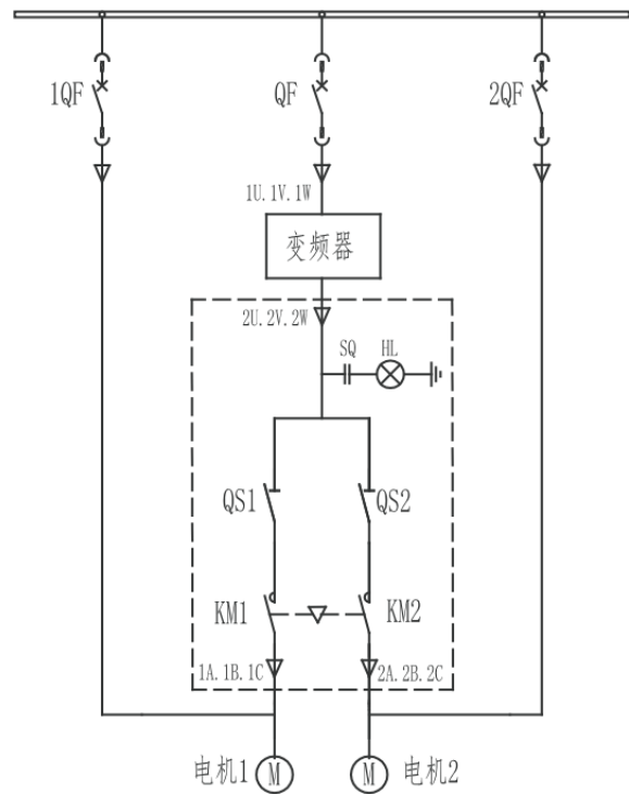
图3.26 自动切换柜一次图
