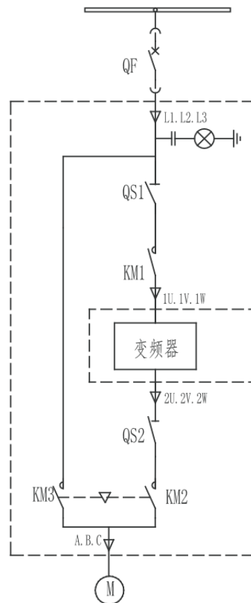
图3.24 自动旁路柜一次图
