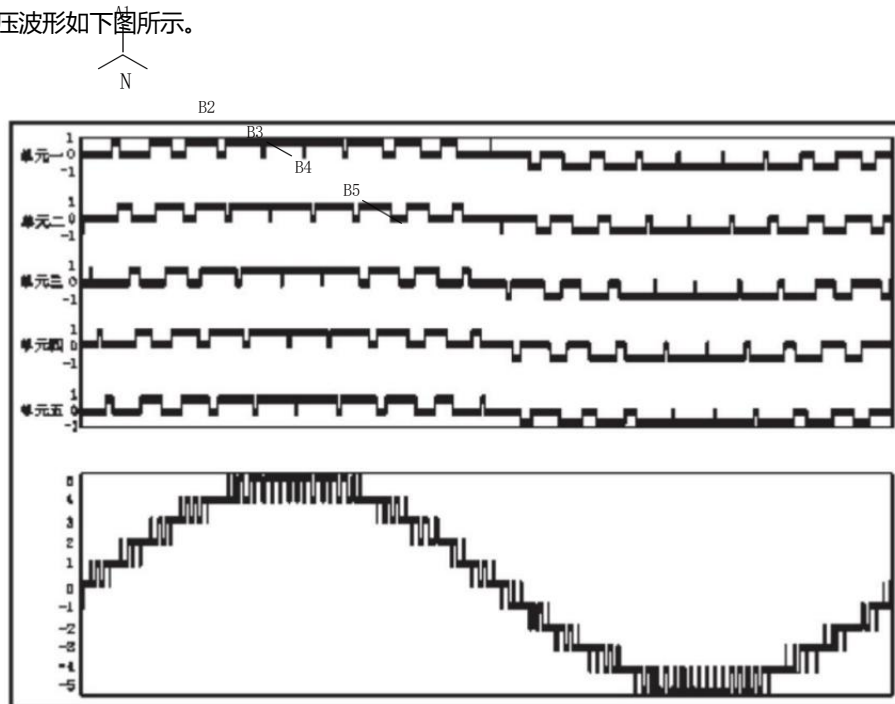
图3.5 6kV变频器输出相电压波形
