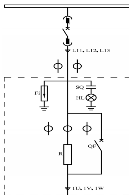
图 3.22 启动柜一次图
