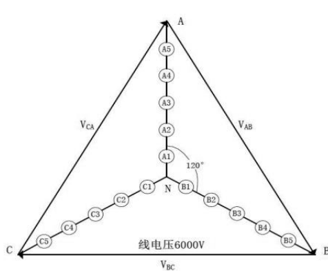
图6.5 5级变频器无旁路示意图
