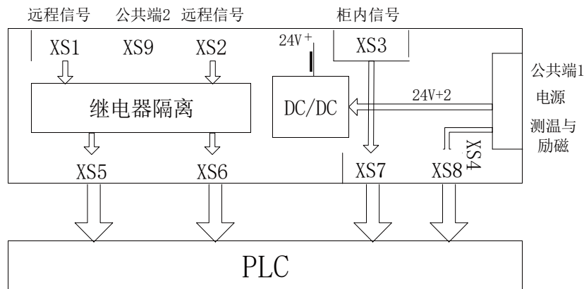
图3.8 接口上板原理框图
