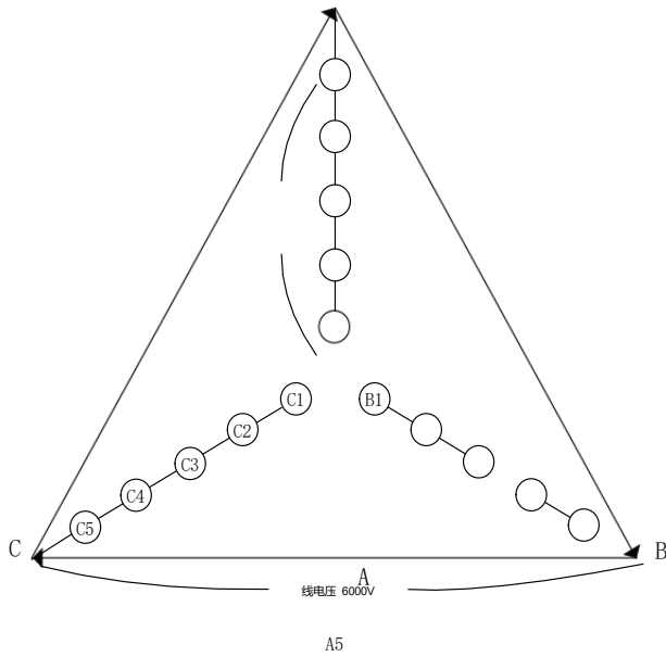
图3.3 6kV变频器单元电压叠加图
